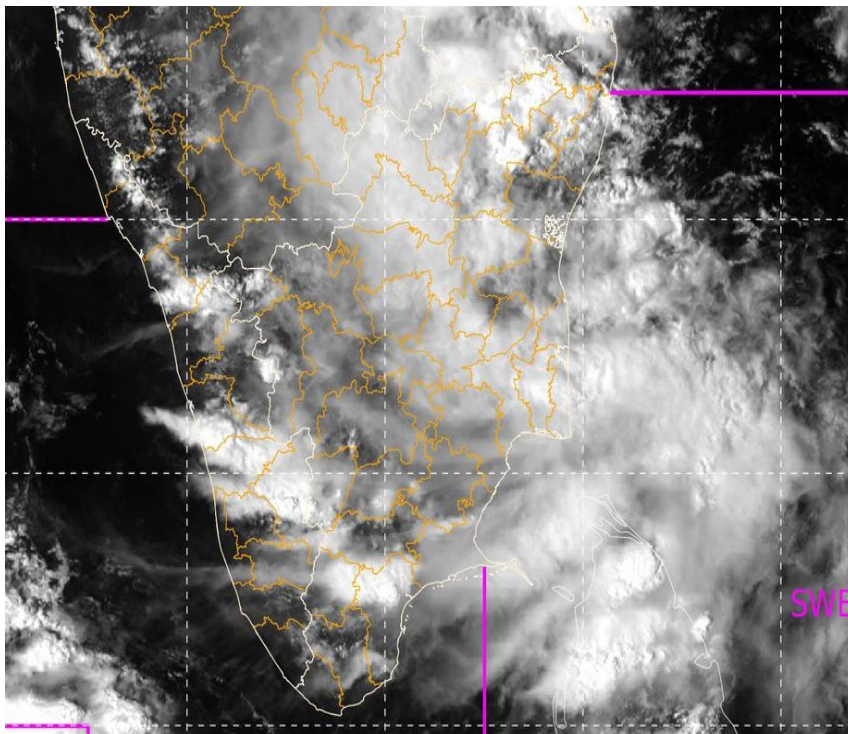
Satellite image at 1426 IST of 05.10.2021
