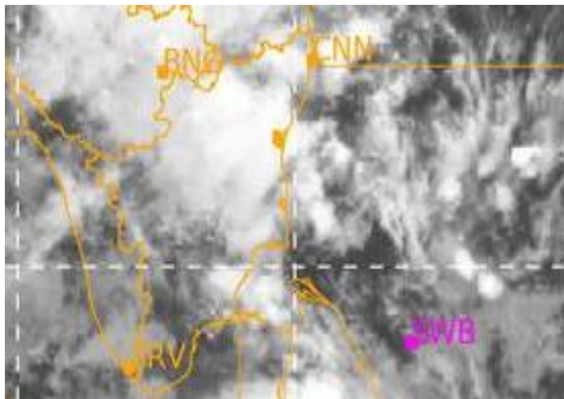
Satellite image at 1730 IST of 29.10.2021
